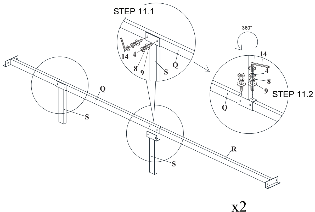
STEP 11 / ÉTAPE 11
