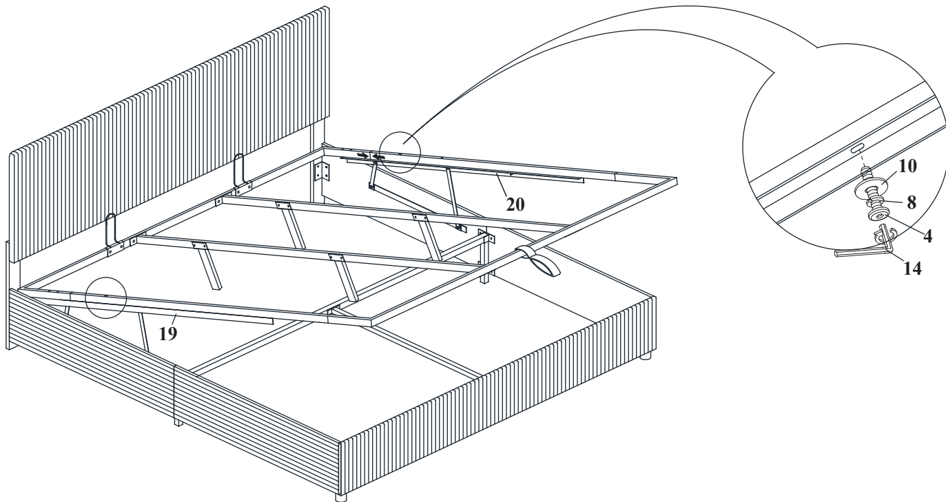
STEP 17 ÉTAPE 17
