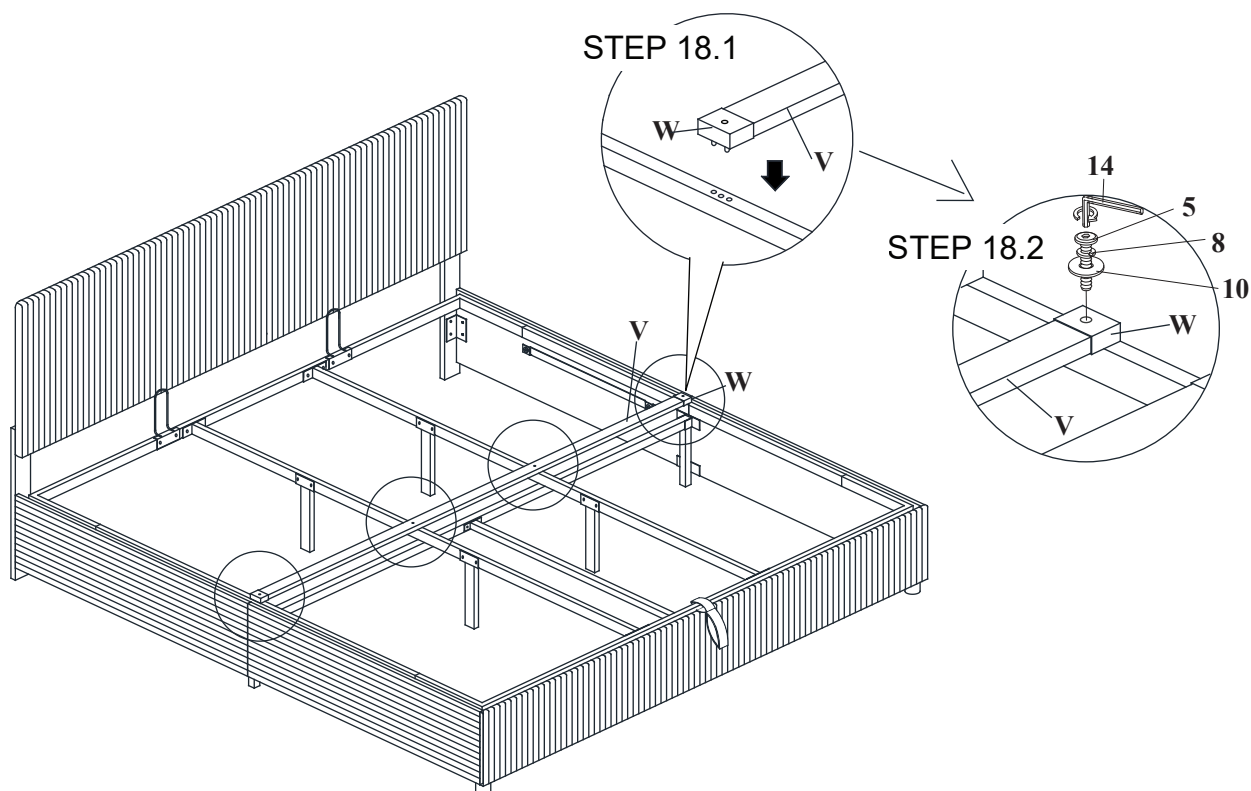
STEP 18 / ÉTAPE 18
